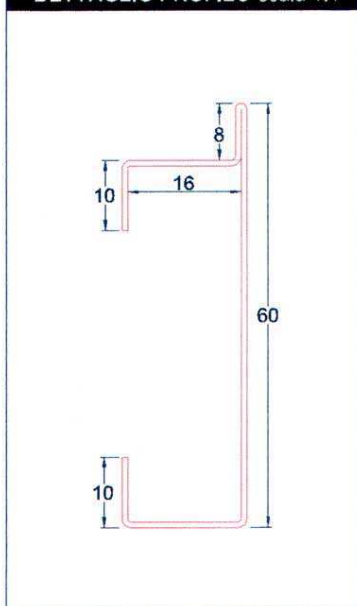
DETTAGLIO PROFILO scala 1:1
