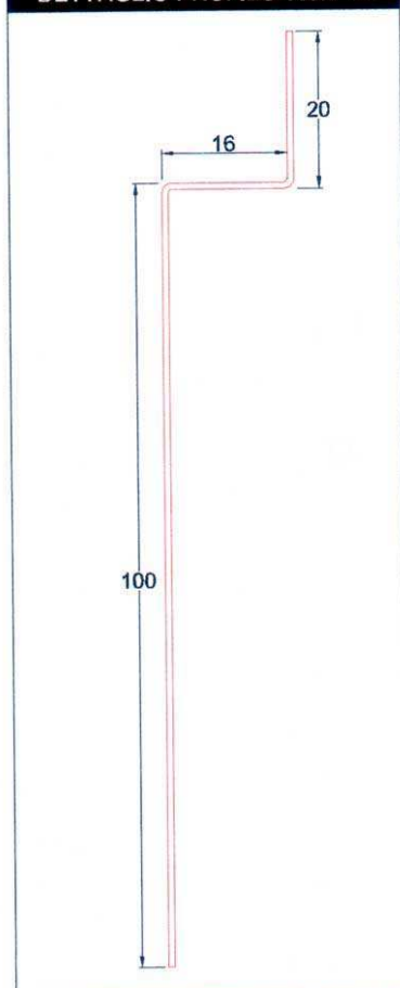
DETTAGLIO PROFILO scala 1:1
